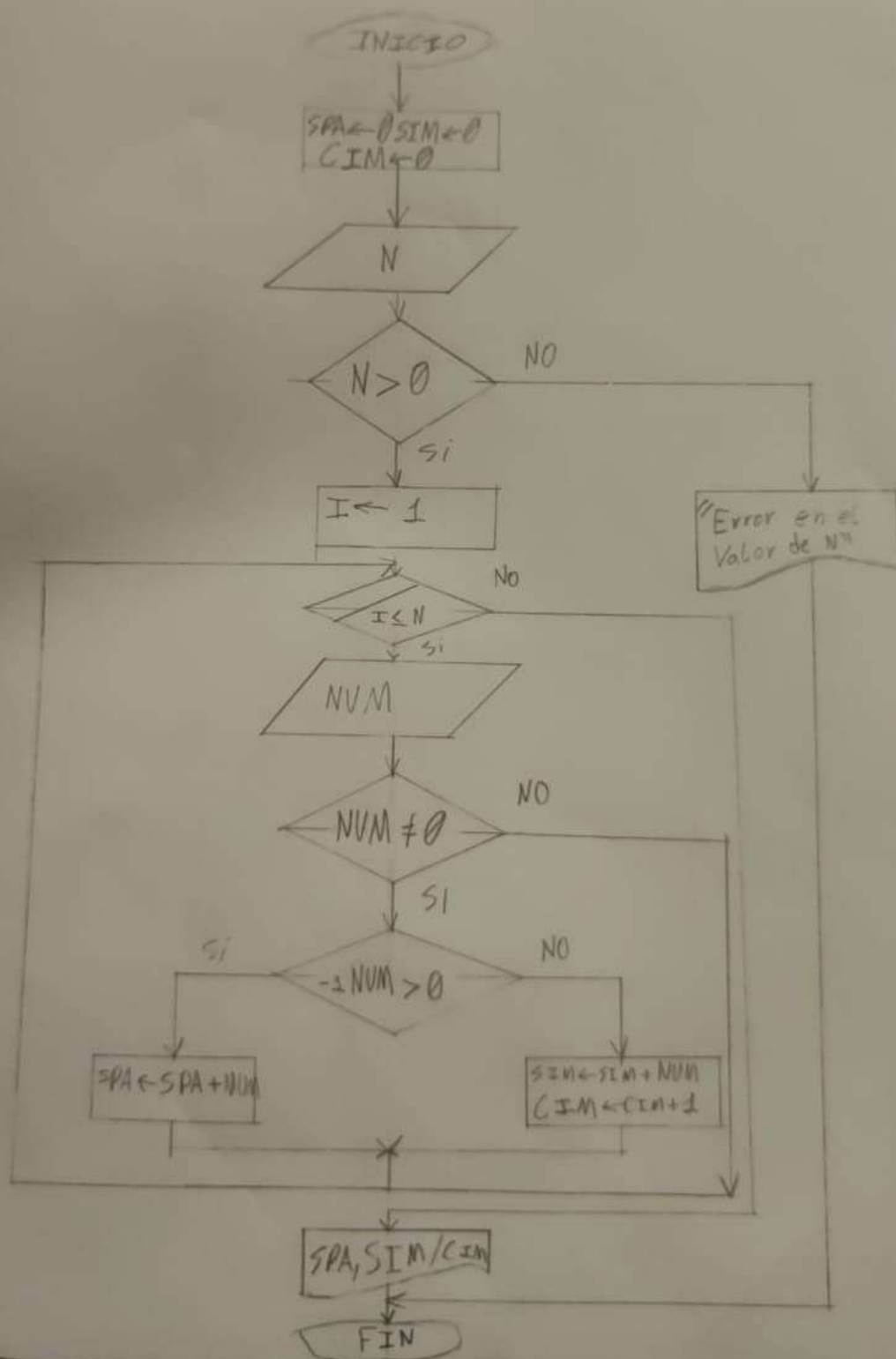
Diagrama de Flujo 3.10
