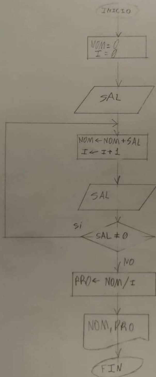
Diagrama de Flujo 3.6
